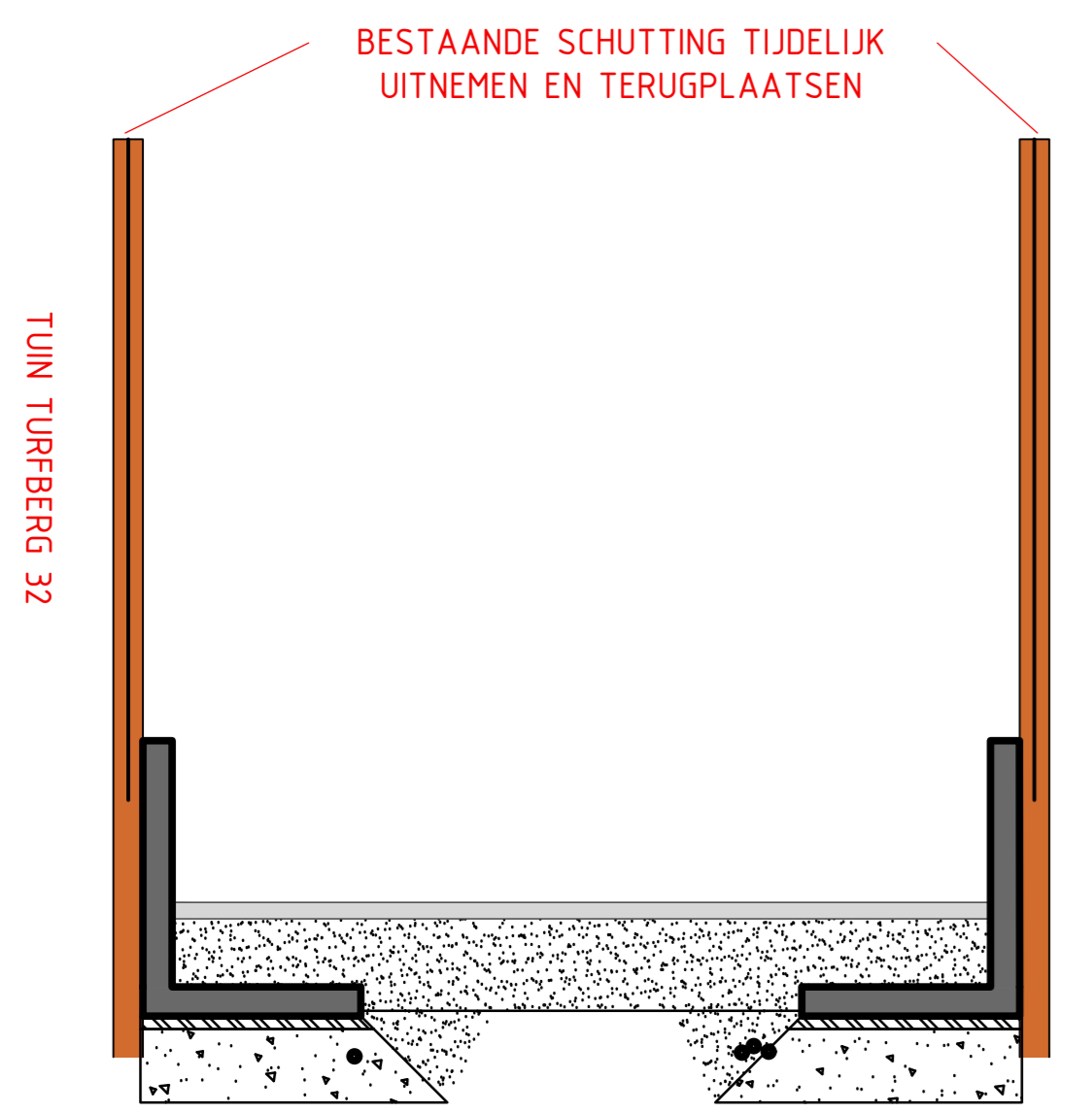
DOORSNEDE - 2 ZIJDEN KEERWAND GRENZEND AAN PARTICULIERE TUIN SCHAAL 1:20
