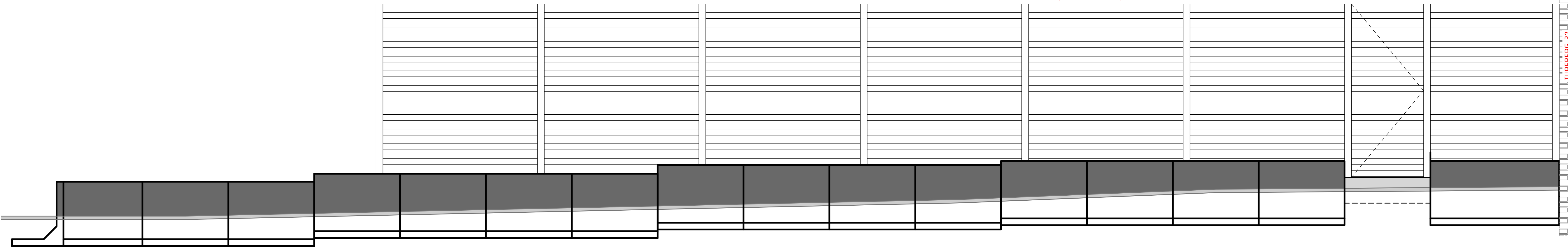
DOORSNEDE EN AANZICHT - KEERWAND GRENZEND AAN TUIN TURFBERG 32 SCHAAL 1:20
