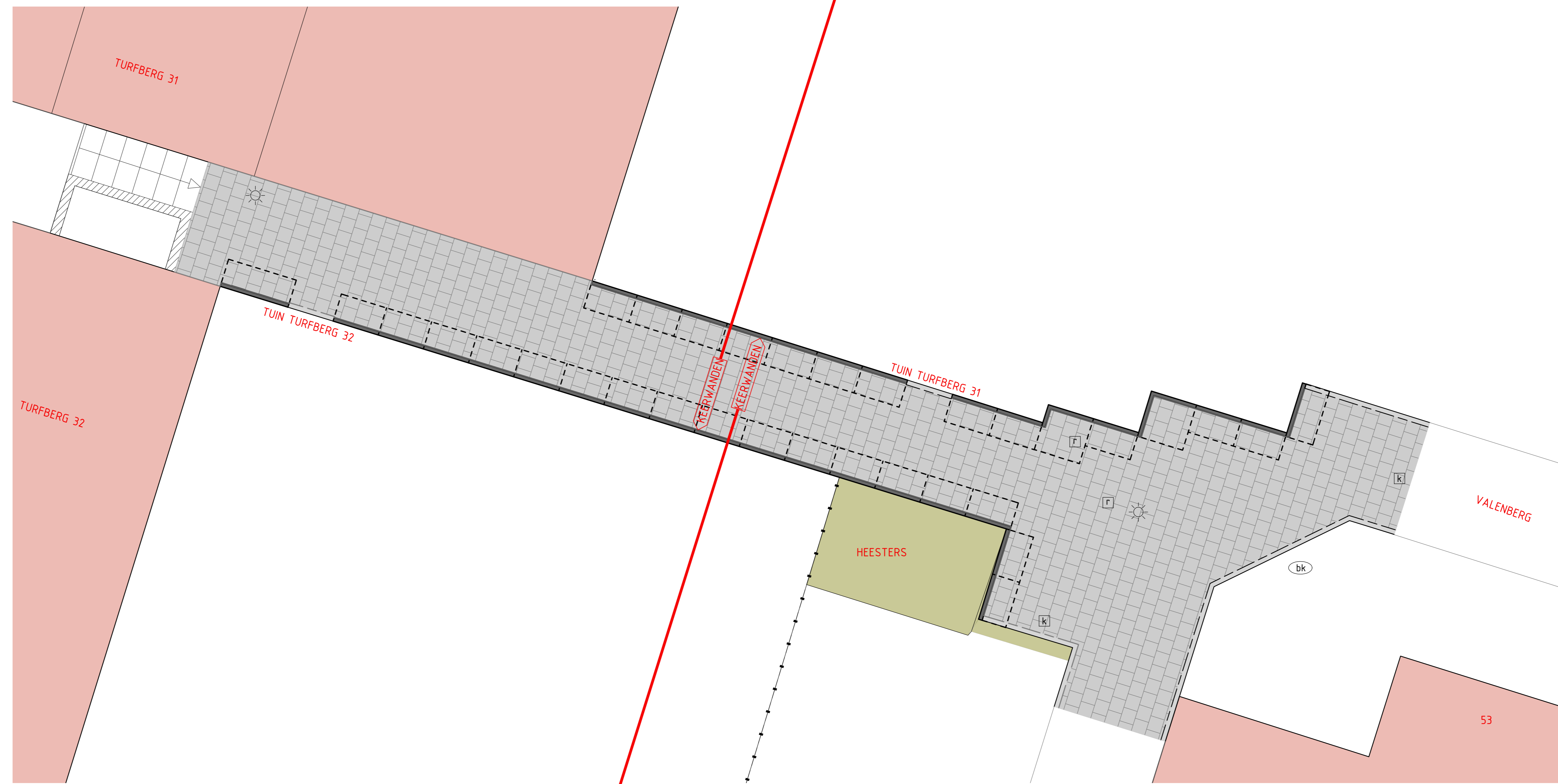
LOCATIE B-06 T.P.V. TURFBERG 31-32 - NIEUWE SITUATIE SCHAAL 1:50
