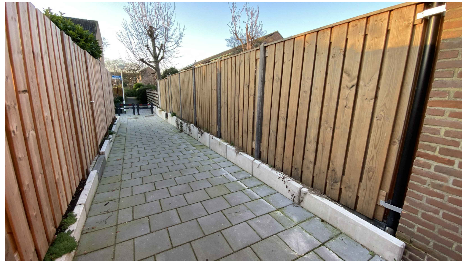
VOORBEELD - 2 ZIJDEN KEERWAND GRENZEND AAN PARTICULIERE TUIN, GETRAPPT AANGEBRACHT
