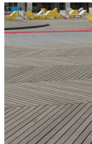
Plein als meubelstuk van het winkelhart. De vloer van hoogwaardig beton refereert naar een plankenpatroon van een houten vloer. het horizontale plein krijgt een hoogteverschil door aflopende straten waardoor een zitrand ontstaat.
