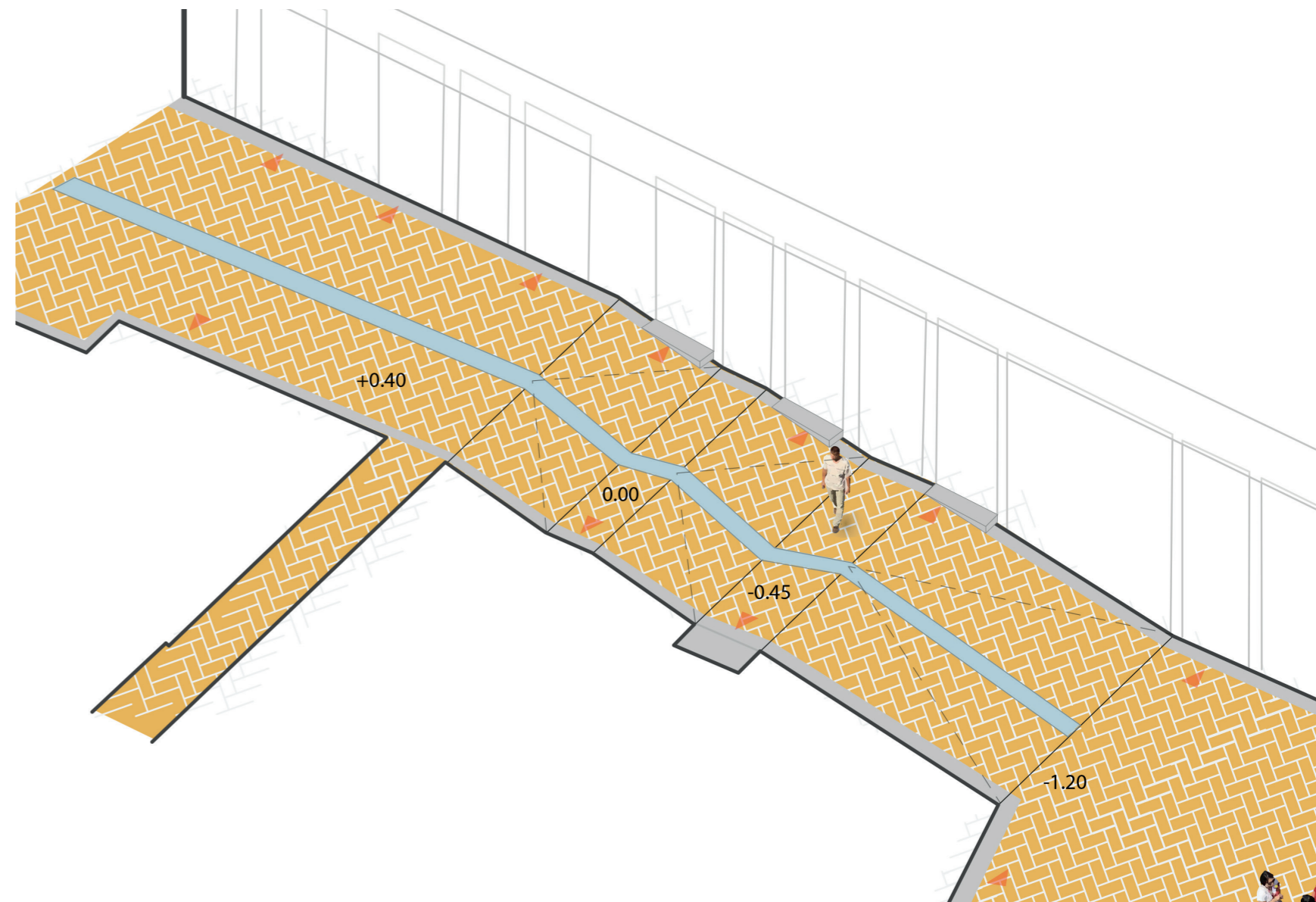
Principe hoogteverschillen Een afwisseling tussen plateau en hellingbaan voor optimale toegankelijkheid met een hellingspercentage volgens de richtlijnen van het ASVV
