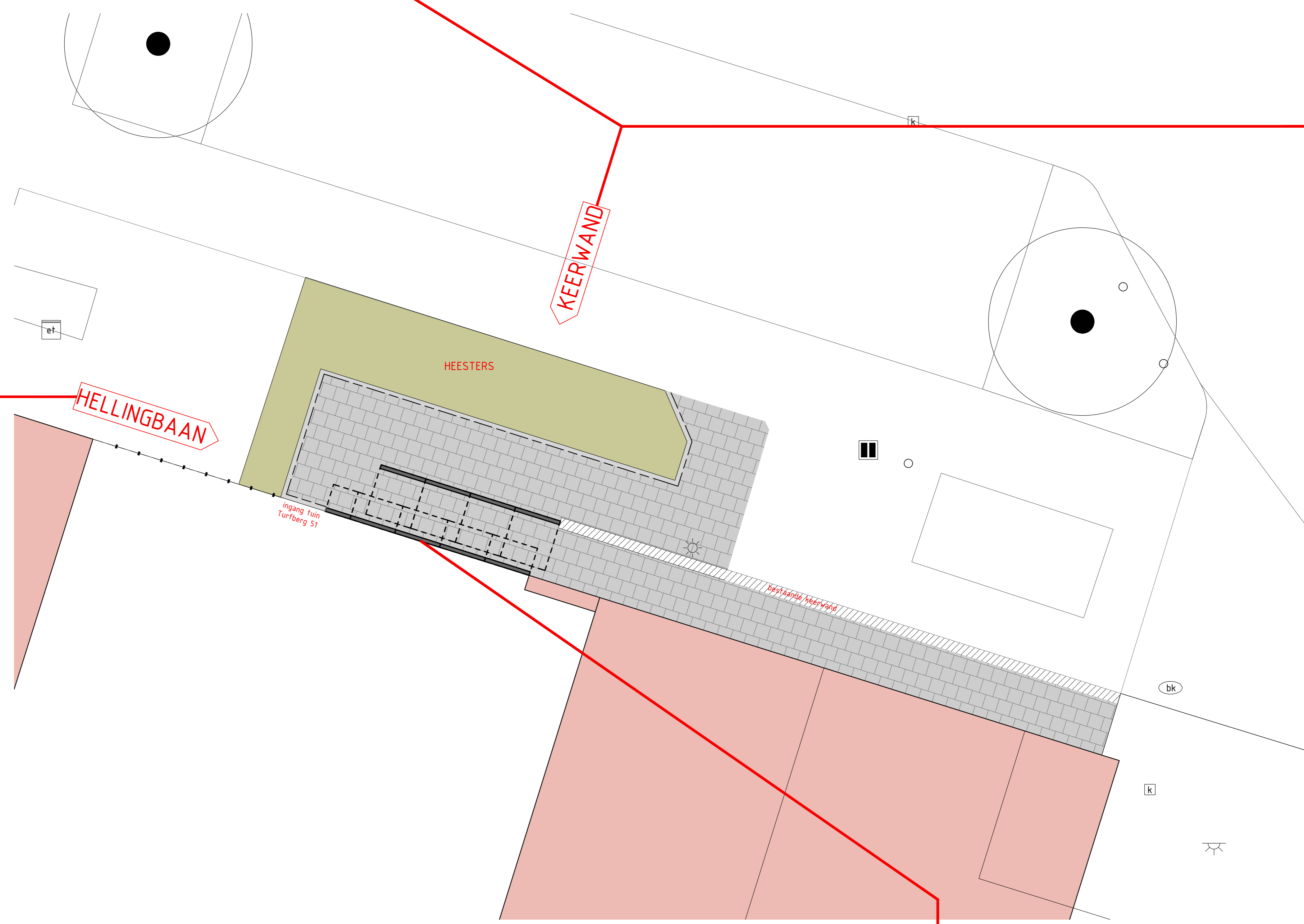
LOCATIE B-03 T.P.V. TURFBERG 51 - NIEUWE SITUATIE SCHAAL 1:50
