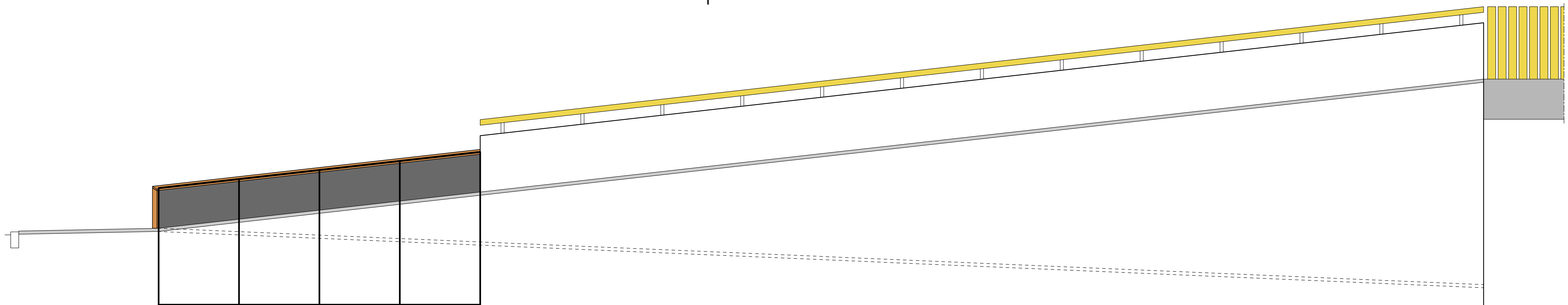
DOORSNEDE EN AANZICHT KEERWAND MET HOUTEN DEKSLAAF SCHAAL 1:20
