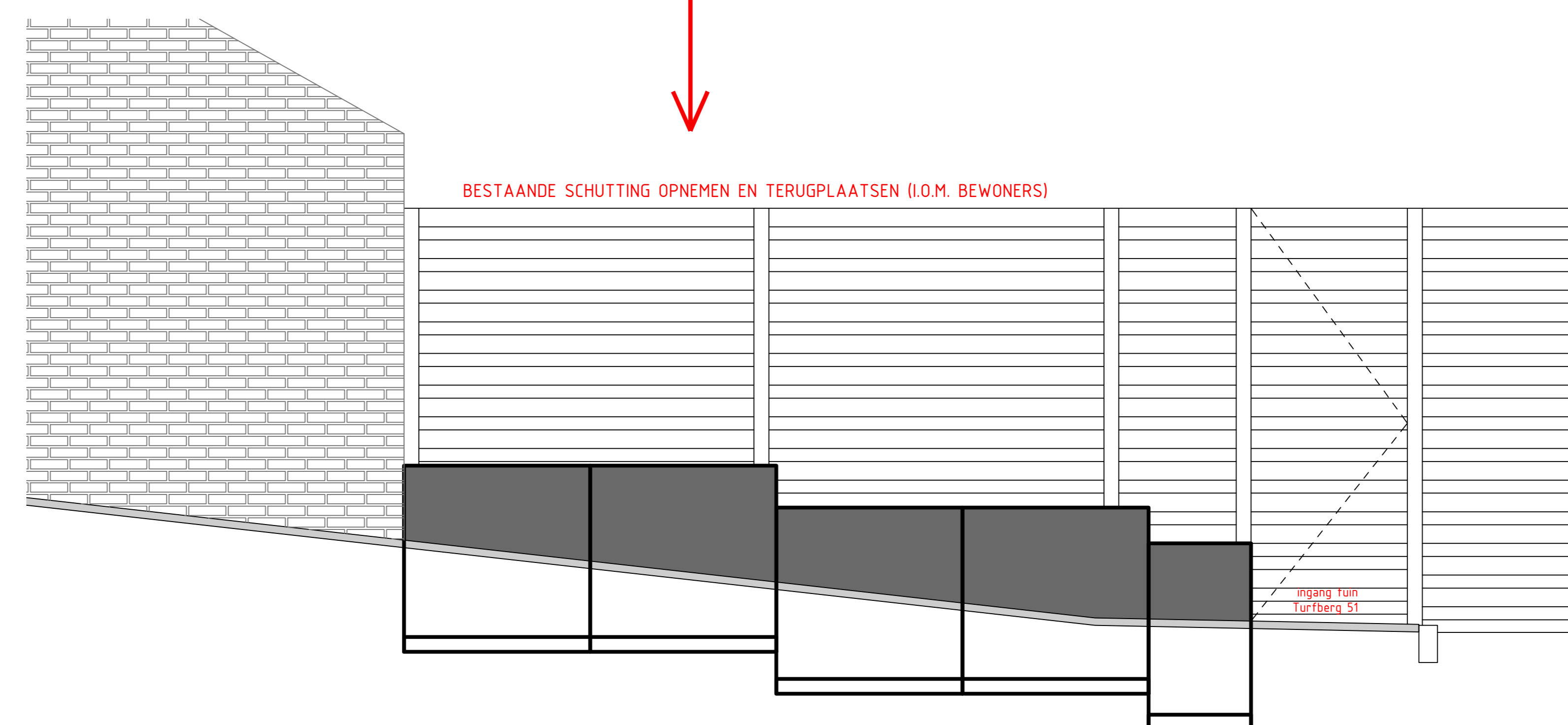
DOORSNEDE EN AANZICHT KEERWAND GRENZEND AAN TUIN TURFBERG 51 SCHAAL 1:20
